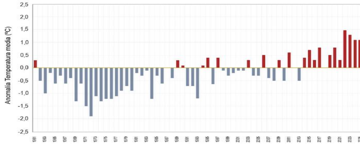
Figura 16.5: Anomalías de temperatura de 2025 en la España peninsular desde 1961 con respecto al periodo de referencia 1991-2020
