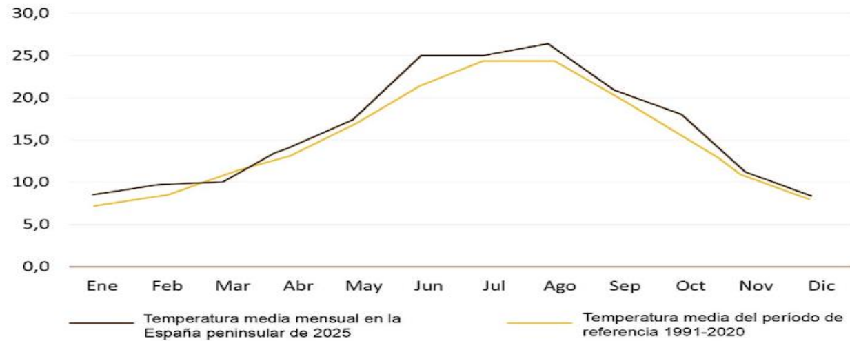
Figura 16.6: Temperatura media mensual en la España peninsular de 2025 y temperatura media del periodo de referencia 1991-2020
